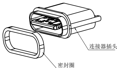
密封圈
